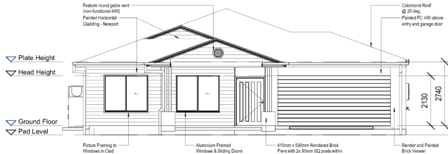
Elevation 1
