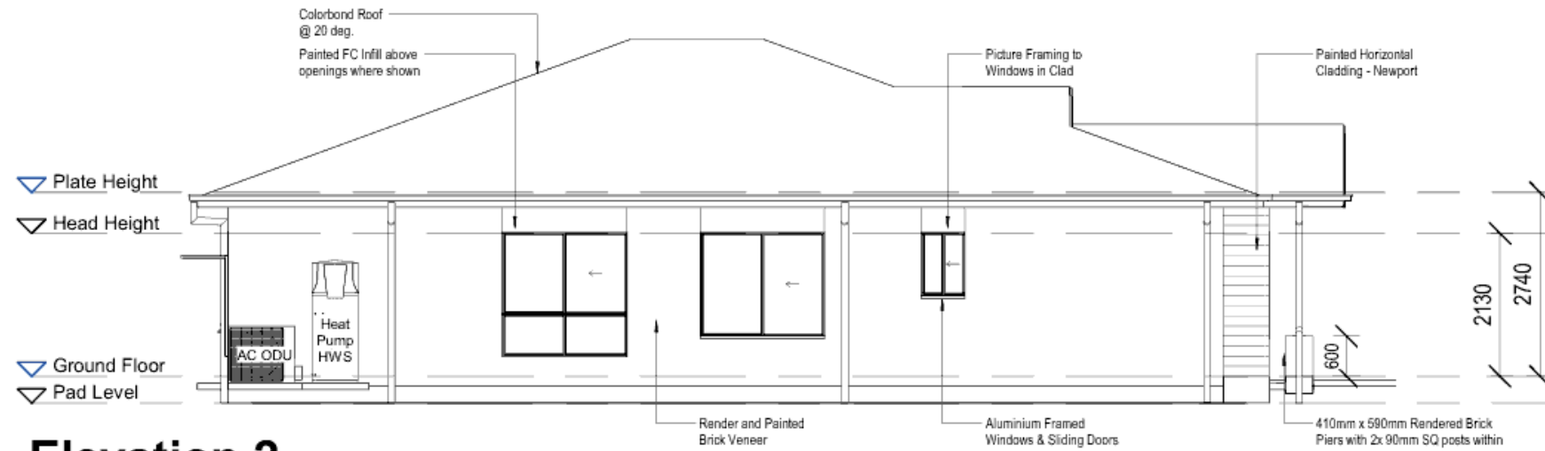
Elevation 2
