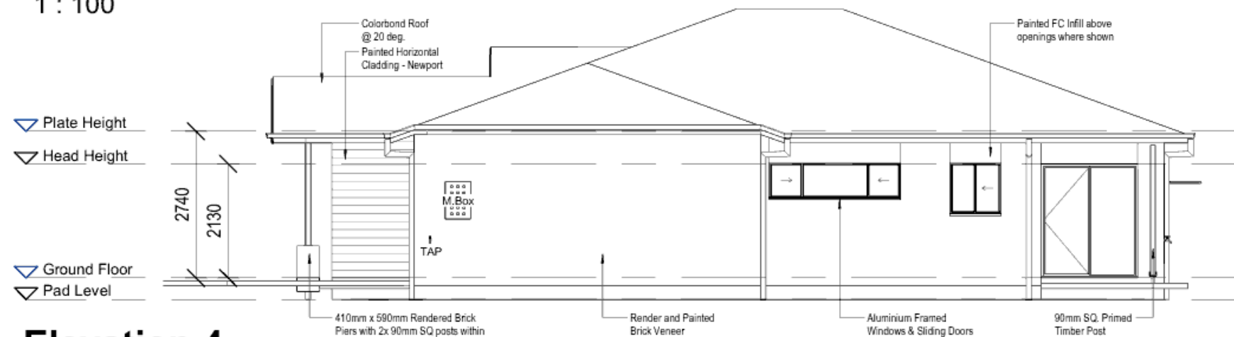
Elevation 4
